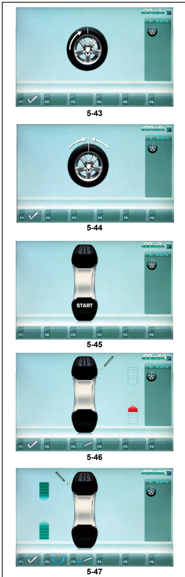
Рис. 5-43 ОПТИМИЗАЦИЯ “OP.7”
