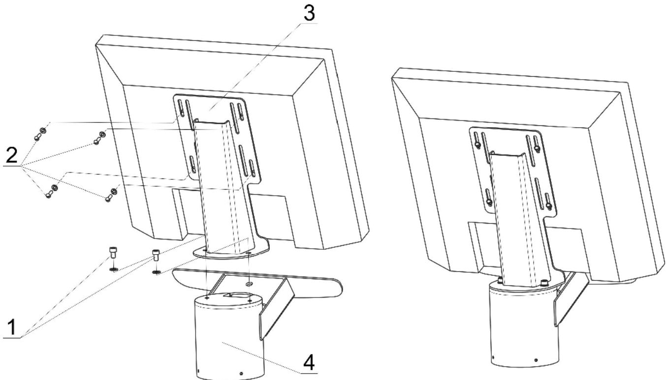
Рисунок 4.7 - Установка монитора
